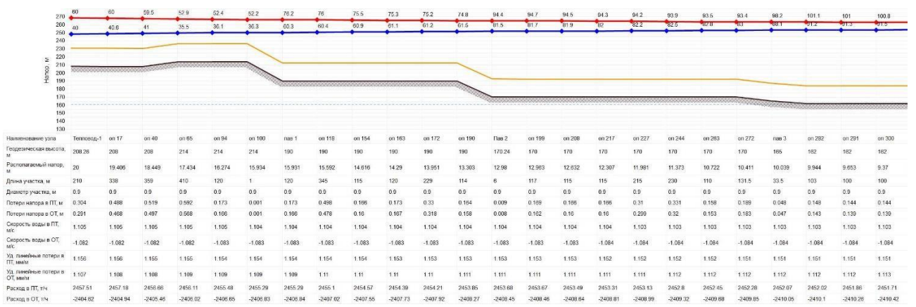
Рис. 4.7. Пьезометрический график при проектировании тепловода \varnothing 900
