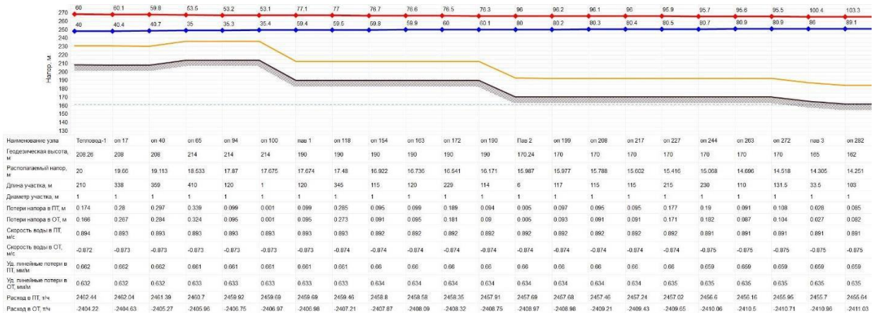
Рис. 4.8. Пьезометрический график при проектировании тепловода \varnothing 1000
