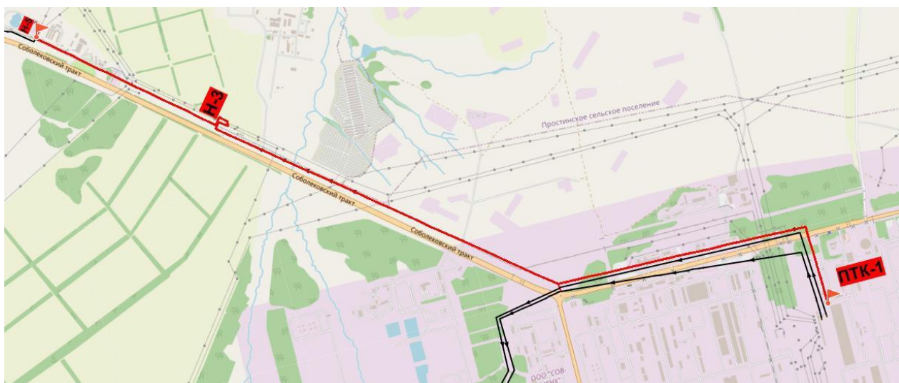
Рисунок 4.2. Магистральный тепловод Город – 2
