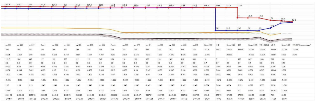
Рис. 4.7. (продолжение) Пьезометрический график при проектировании тепловода \varnothing 900
